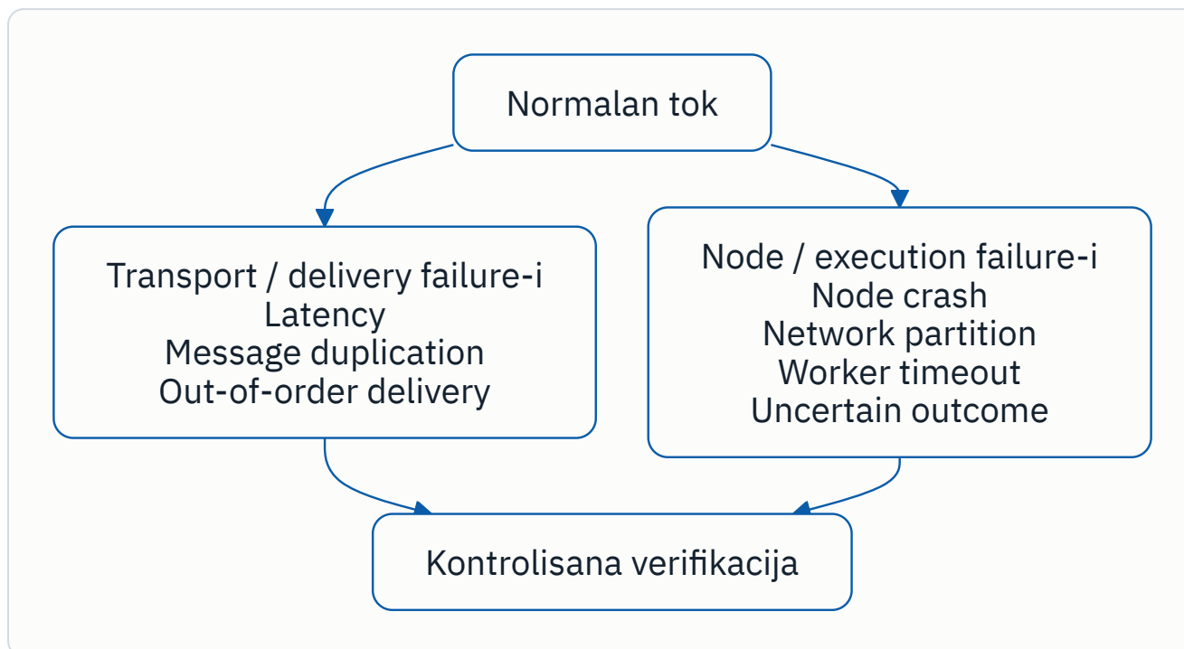
Slika 9. Referentni failure model koji simulatori mogu kontrolisano da izazovu.
